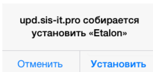
Рисунок 5 - Установка версии
