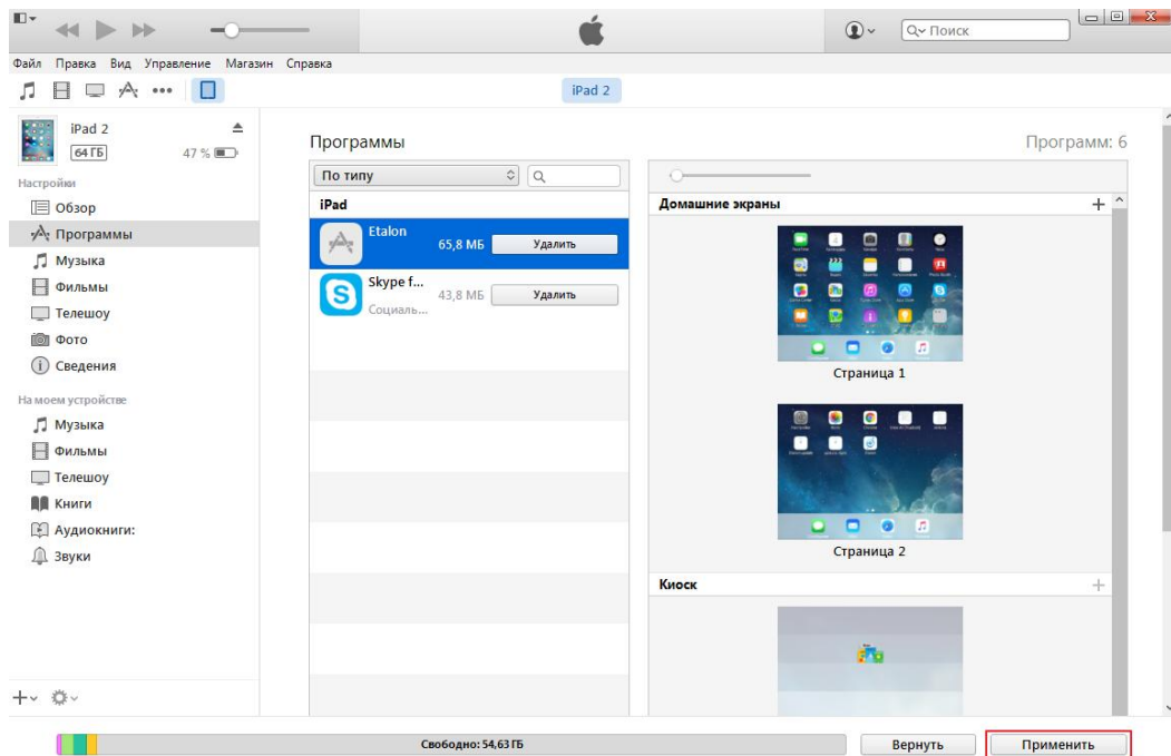
Рисунок 3 - Установка приложения
