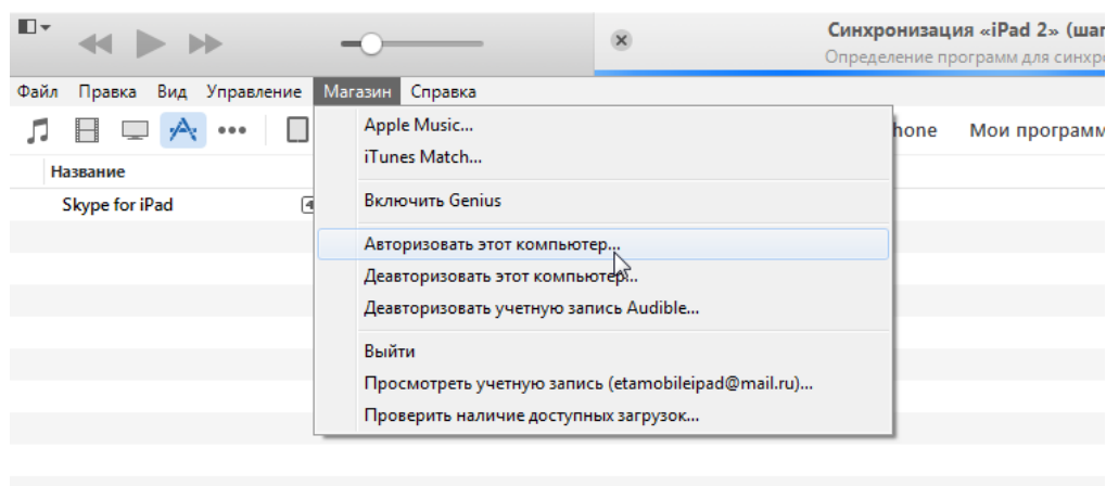
Рисунок 1 - Авторизация компьютера
