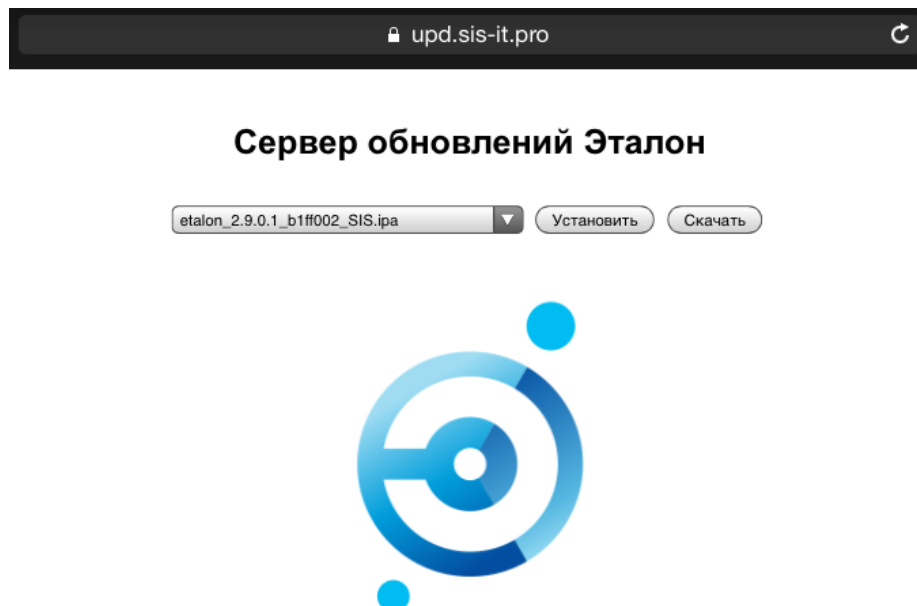
Рисунок 4 - Сервер обновлений
